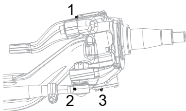
Figura 61: Puntos de lubricación del eje delantero del PACCAR FX-20
