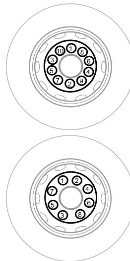
Figura 63: Ruedas de disco centradas por cubo
