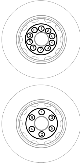
Figura 64: Ruedas disco centradas por espárragos
