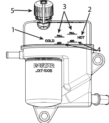
Figura 62: Depósito de dirección hidráulica
