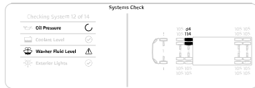
Illustration 10 : Vérification du système avec TPMS
