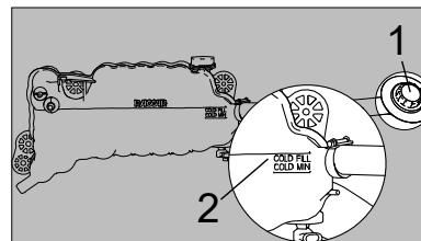
Illustration 62 : Réservoir d'équilibre de liquide de refroidissement monté sur cloison
