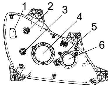
Illustration 66 : Ensemble de phares T680
