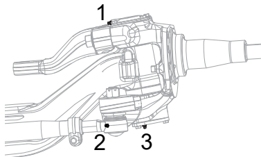
Illustration 60 : Points de graissage pour essieu avant FX-20 PACCAR
