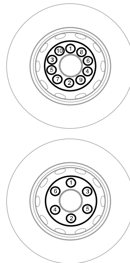
Illustration 70 : Roues à disque centrées par goujons
