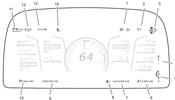
Illustration 18 : Indications sur l'écran
