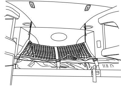
Illustration 5 : Dispositifs de retenue de la couchette supérieure
